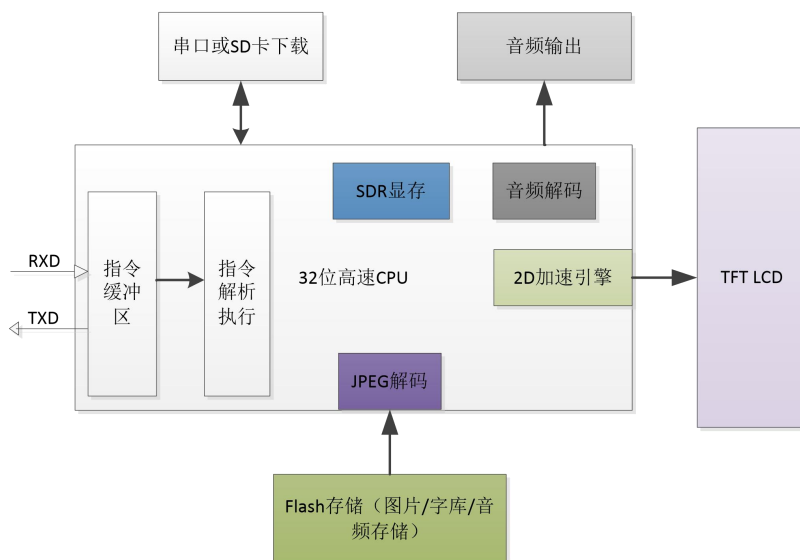
图 11-1 M 系列串口屏内部结构图
